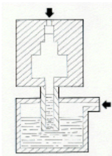
Figuur 8.2 Schematisch overzicht coquille gieten (lage-druk)
