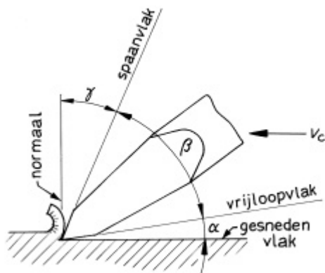
figuur 4 Hoeken, spaanvlak en vrijloopvlak bij een platte beitel
