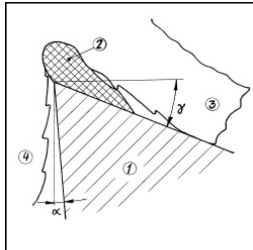
figuur 1: Vorming van een valse snijkant. 1. beitel, 2. valse snijkant, 3. spaan, 4. oppervlaktegesteldheid, \alpha vrijloophoek, \gamma spaanhoek
